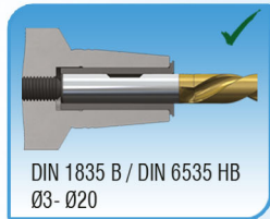
Pens ile sıkma Clamping with reducing arbor (Düşük tork ve salgı) (low torque and roun-oul)
